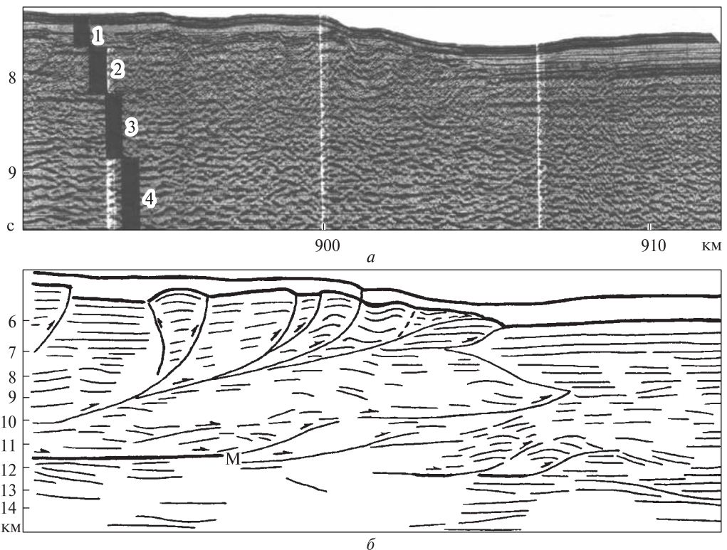
Рис. 3. Фрагмент профиля МОГТ 1 с двумя АТЗ первого типа в слое 2 между пикетами 899–902 км. а — временной разрез, б — глубинный разрез. Остальные обозначения см. в подписи к рис. 2.
