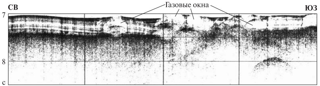
Рис. 5. Фрагмент профиля НСП (5 на рис. 1) на севере котловины Тускарора с газовыми окнами в неоген-раннечетвертичных осадках вершины Камчатского контурного мегафана
