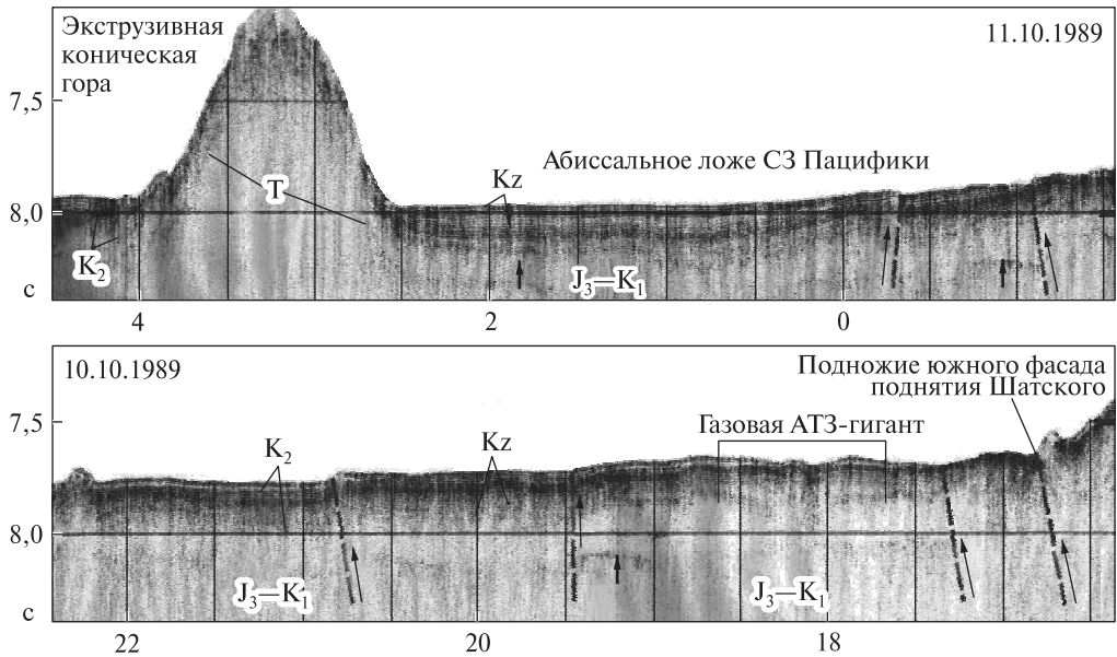
Рис. 4. Фрагмент профиля НСП 114 с Гагаринским АТЗ-гигантом, газовыми окнами в кровельных траппах, разломами и смещениями по ним — пунктир со стрелкой. Вертикальный масштаб в секундах двойного пробега здесь и на рис. 5—8. Вертикальные линии — полчасовые марки времени (здесь и на рис. 5—8). Стратиграфия разреза по [1, 3]. Координаты АТЗ в тексте
