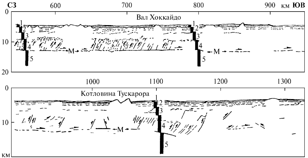
Рис. 2. Глубинный разрез МОГТ 1 близ разлома Тускара и профиля ГСЗ ИФЗ РАН 1—0, один из лучших по геологической информативности в океане [2]. Координаты: профиля — 41^{\circ} 45.9' с. ш., 150^{\circ} 12.4' в.д., конца профиля — 35^{\circ} 59.3' с.ш., 153^{\circ} 01.8' в.д. геофизические слои 1—5; М — подошва аллохтонной океанической коры (слои 1—4) и деколlement СЗ плиты Пацифики; Наклонные линии со стрелками — чешуйчатые надвиги и смещения по ним. Временной разрез полностью приведен [27]
