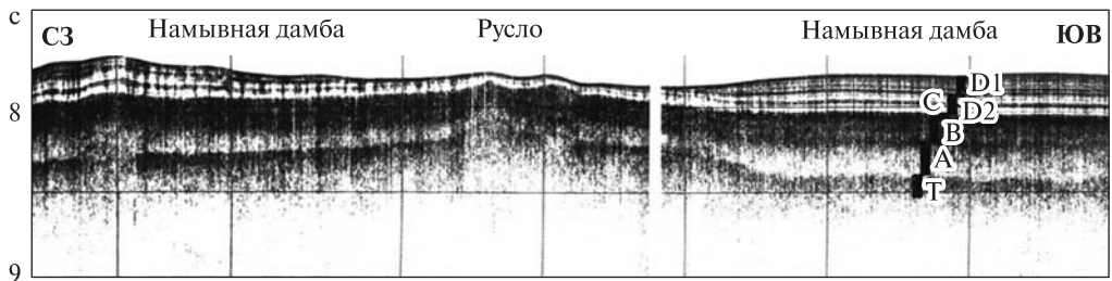
Рис. 6. Фрагмент профиля НСП (6 на рис. 1) на востоке котловины Тускарора с газовыми «нитями» в неоген-раннечетвертичных осадках (толща D или D1, 2 ) долины Камчатского мегафана, обвалованной намывными дамбами
