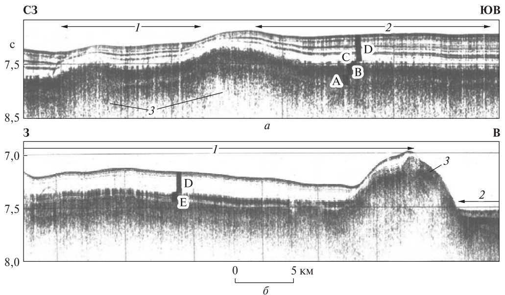
Рис. 8. Фрагменты профилей НСП. Условные обозначения к стратиграфии чехла см. рис. 7. а — проф. 8, а на рис. 1. 1 — конседиментационные деформации неоген-четвертичного срыва слоев 1—4 (центральная часть котловины Тускарора) и многочисленные газовые столбы и «нити» в мезокайнозойском чехле, включая маломощный горизонт С; б — проф. 8, б на рис. 1. с газовыми столбами и «нитями» в контрастном сейсмокомплексе Е (вероятно прибрежные осадки позднего палеогена по аналогии с скв. 192 [19] близ северного окончания поднятия Шатского. 1 — восточная лопасть Камчатского мегафана, 2 — эрозионная долина, 3 — молодой постседиментационный экструзивный холм (протрузия гранитов)?
