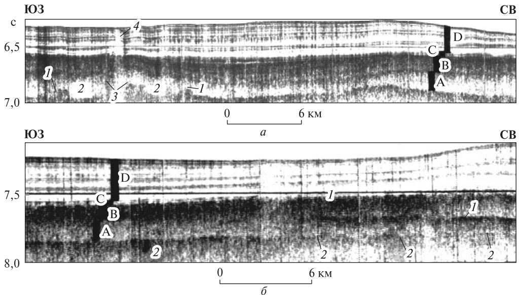
Рис. 7. фрагменты профилей НСП: 1 — барьерный риф; 2 — внутренняя лагуна; 3 — центральный риф. А—D — стратиграфия чехла: А — карбонатная толща поздней юры-раннего мела; В — позднемеловой опактовый горизонт пестрых кремней и глин; С — пестрые лессы пенеплена Пацифики; D — контуриды и турбидиты Камчатского контурного мегафана (здесь и на рис. 8); а — проф. № 7 а на рис. 1 в котловине Тускарора с газовым столбом (4), «нитями» и миниатоллом в шельфовом карбонатном бассейне позднего Тетиса. б — проф. № 7 на рис. 1 близ основания западного склона поднятия Шатского с газовыми «нитями» и ярусным строением финальных траппов (1, 2) мезозойской трапповой формации в карбонатном матрикс позднего эпиконтинентального Тетиса
