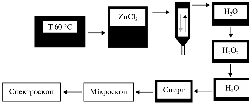
Рис. 1. Схематичне зображення етапів підготовки проб та досліджень МП у складі донних відкладів, що виконувались в ДНУ «МорГеоЕко-Центр»: сушка, сепарація в розчині хлористого цинку, попередній відбір виділеної речовини, тонкий відбір на роздільній воронці, промивка в дистилляті, відстоювання в пероксиді водню, промивка в дистилляті, знежирювання в спирті, мікроскопічні дослідження сухої речовини та верифікація результатів на Раман-спектроскопі
