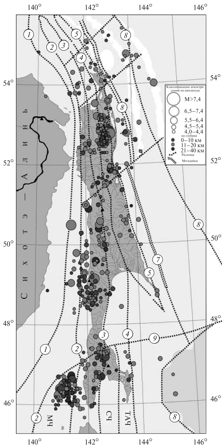
Карты эпицентров землетрясений с M \geq 4 (1906–2005 гг.), региональных разломов и основных тектонических структур Сахалина. Региональные разломы: 1 – Восточно-Сихотэ-Алиньский, 2 – Западносахалинский, 3 – Центральносahalинский, 4 – Хоккайдо-Сахалинский, 5 – Северо-Сахалинский, 6 – Трехбратский, 7 – Пограничный, 8 – Восточносahalинский, 9 – Стародубский. Коровые аллохтонные пластины: Западно-Сахалинская – между разломами 1 и 3; Восточно-Сахалинская – между разломами 3 и 8. Коровые аллохтонные чешуи: МЧ – Монеронская, СЧ – Сусунайская, ТАЧ – Тонино-Анивская. Антиклинории: Западносахалинский – между разломами 2 и 3; Восточносahalинский – между разломами 3 и 8; Центральносahalинский синклиний – на Северном Сахалине между разломами 3 и 4
