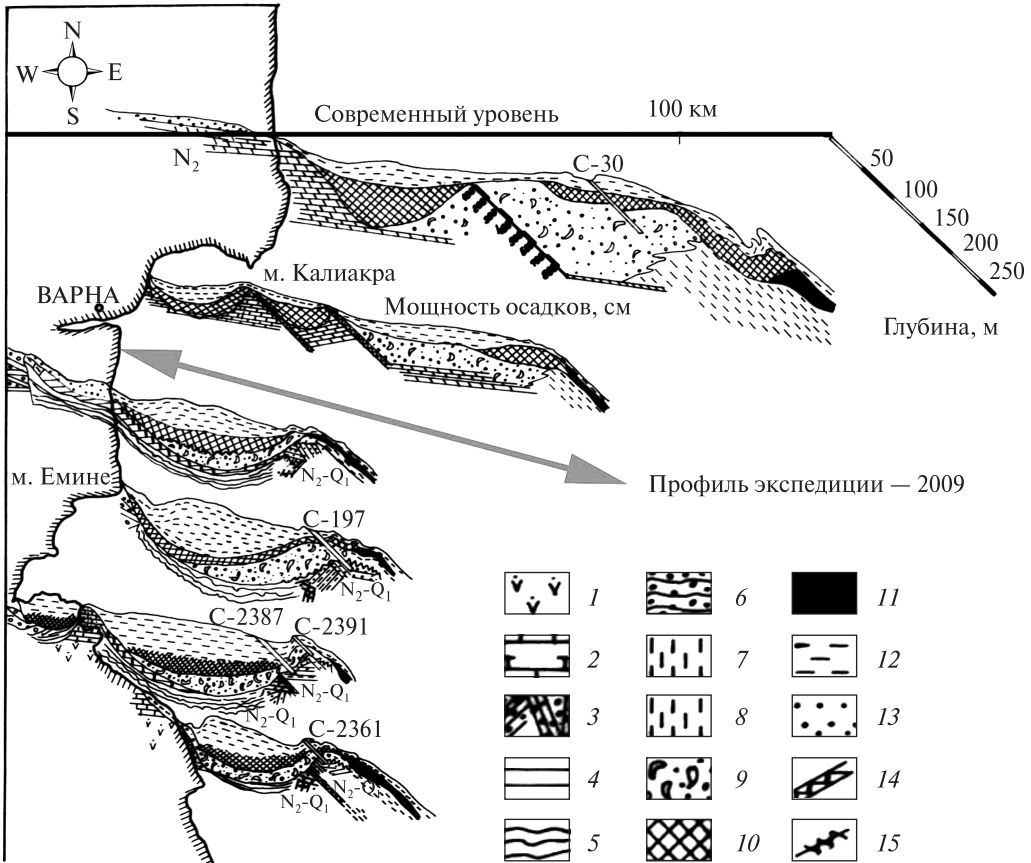
Рис. 4. Схематические геологические разрезы плейстоцена — голоцена. С-2387 — номер скважины: 1 — вулканогенно-осадочный комплекс; 2 — сарматские известняки; 3 — прибрежноморские фации плейстоцена и верхнего плиоцена; 4 — песчаные глины с чаудинской фауной; 5 — развитие континентальных и лиманных осадков; 6 — континентальные русловые фации; 7 — карпатские и новоэвксинские осадки; 9 — прибрежноморские осадки новоэвксина; 10 — древнечерноморские илы; 11 — сапропелевые илы; 12 — новочерноморские илы; 13 — пески; 14 — разломы; 15 — эрозионная граница
