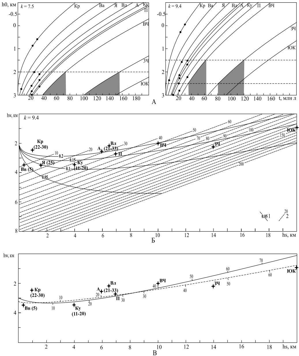
Рис. 3. Определение возраста и эволюции погруженного состояния субокеанических впадин.
