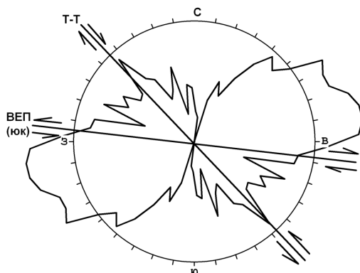
Рис. 8. ДПР верхнекимерийского структурного яруса по подошве терригенного комплекса сеноманского яруса - K_2s (lg шкала, 5^\circ классы)
