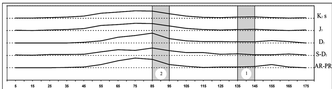
Рис. 9. Гистограммы простираний разломов отдельных структурных ярусов глубинных уровней разреза СЗ шельфа Черного моря
