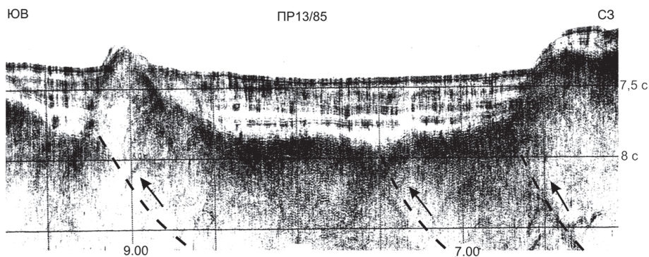
Рис. 6. Фрагмент профиля НСП 13/85 в котловине Тускарора через раннемиоценовую? моноклинальную гряду, связанную с начальной фазой срыва слоев 1-4 к ЮВ от вала Хоккайдо (НИС "Петас"-1985)
