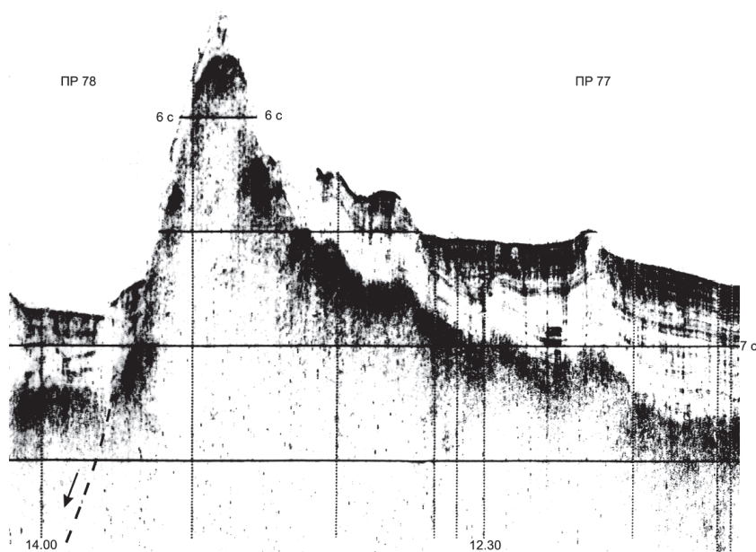
Рис. 8. Профили НСП 77, 78 через южный борт рифтограбена (раздвиг) с экструзивной одиночной горой в зоне разлома Хоккайдо (НИС “Проф. Гагаринский”-1989). Координаты ПК 12.30 (45° 06,14 с.ш., 157° 01,98 в.д.) и ПК 14.00 (45° 12,29 с.ш., 157° 17,90 в.д.)
