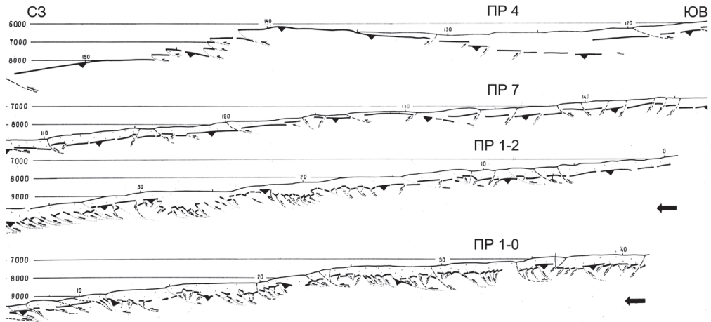
Рис. 3. Глубинные разрезы НСП 4,7 и МОГТ 1-2,1-0 по внешнему склону южной части Курильского желоба (м-б 1:1) [13]. Чешуйчатые надвиги смещают дно и кровлю слоя 2
