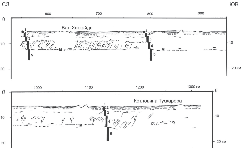
Рис. 1. Глубинный разрез МОГТ 1 [8,19]: 1-5 - геофизические слои, наклонные прерывистые линии со стрелками – чешуйчатые надвиги и смещения по ним. М – деколлемент в подошве океанической коры (слой 1-4). Координаты его начала (41° 45,9 с.ш., 150° 12,4 в.д.) и конца (35° 59,3 с.ш., 153° 01,8 в.д.)
