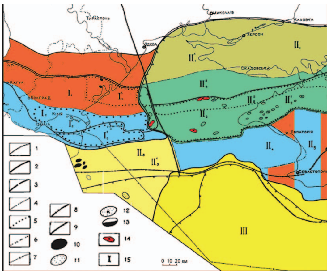
Схема нефтегазогеологического районирования северо-западного шельфа Черного моря. [1, рис. 3.1]
