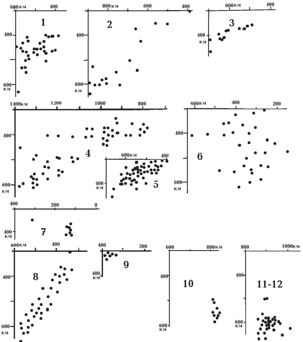
Рис. 6. Глубины гипоцентров глубоких землетрясений вдоль профилей, показанных на рис. 4. Расстояния на горизонтальных осях – от центров глубоководных желобов
