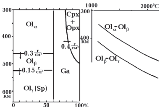
Рис. 2. Минералогия пород мантии при нормальном распределении T и P -условия преобразования оливина (при железистости примерно 13%) в минерал со структурой шпинели. Показаны изменения плотности минералов, стрелки — направление перехода с ростом плотности
